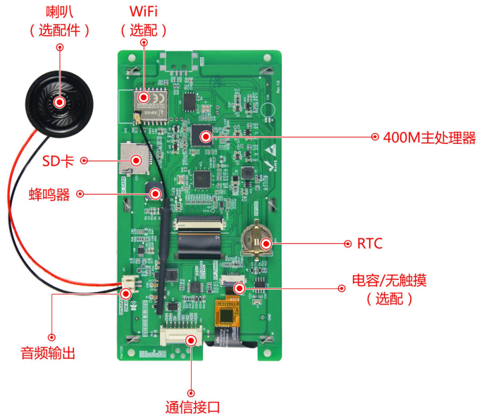
图 1-3 硬件配置图
