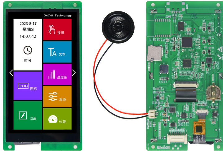
图 1-1 5.5 寸电容触摸参考图
