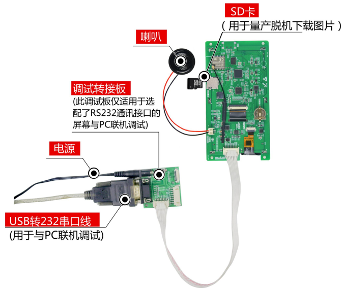
图 1-4 调试工具图
