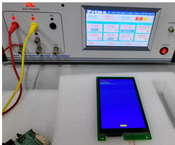
图 4-3 EFT 测试图
