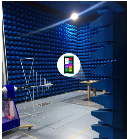
图 4-4 RE 测试图
