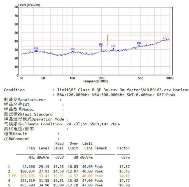
图 4-5 RE 测试水平方向
