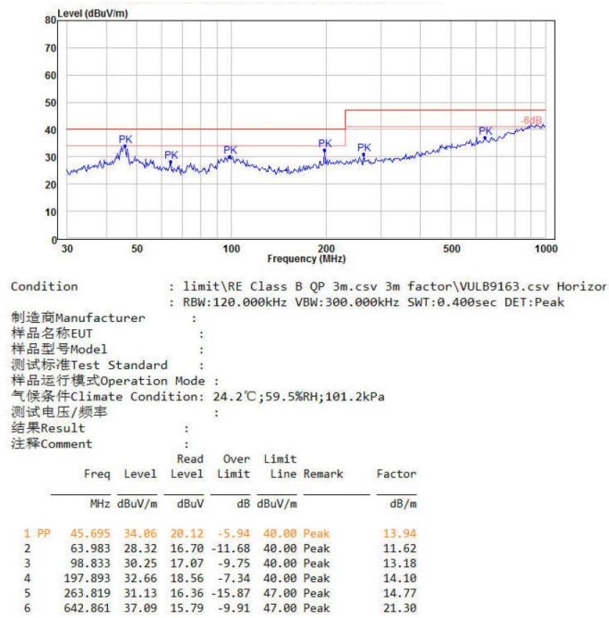
图 4-6 RE 测试垂直方向
